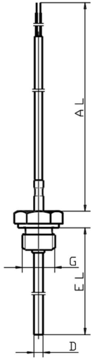
型号: 903730/10
